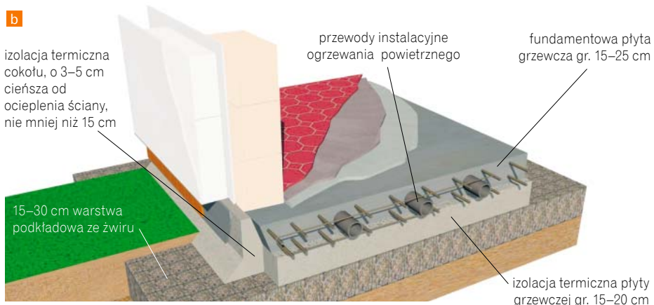
Płyta fundamentowa z ogrzewaniem wodnym (a) (zasilanym np. pompą ciepła) i powietrznym (b)
