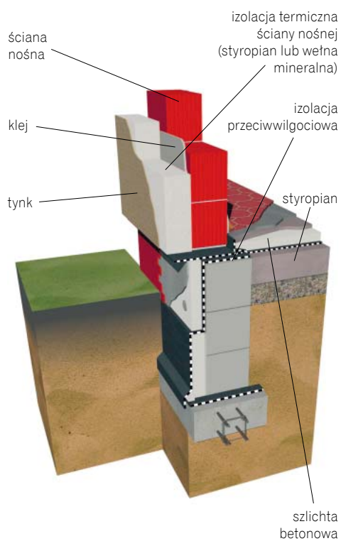
Schemat konstrukcji ściany dwuwarstwowej
