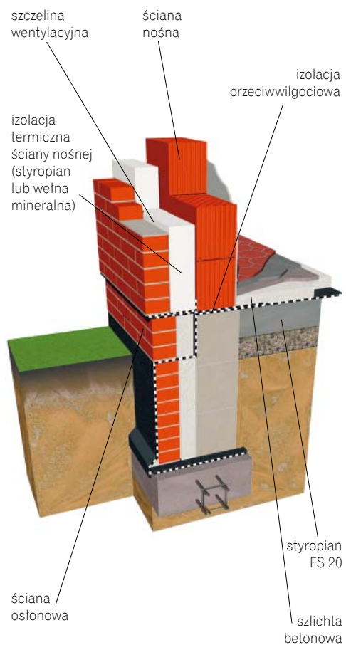
Schemat konstrukcji ściany trójwarstwowej
